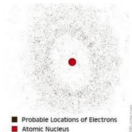
مدل اتم در منطق مکانیک کوانتوم
